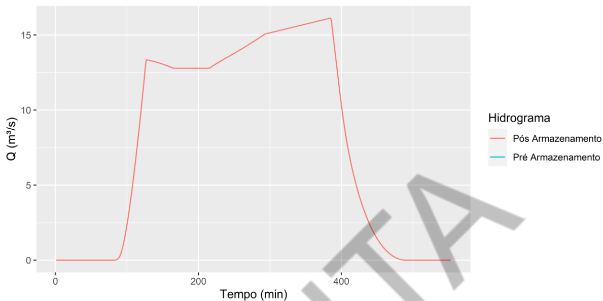
Figura 5 – Hidrogramas de Projeto SMB_01_05, com armazenamento e drenagem na fonte para expansão urbana de 5 anos.
