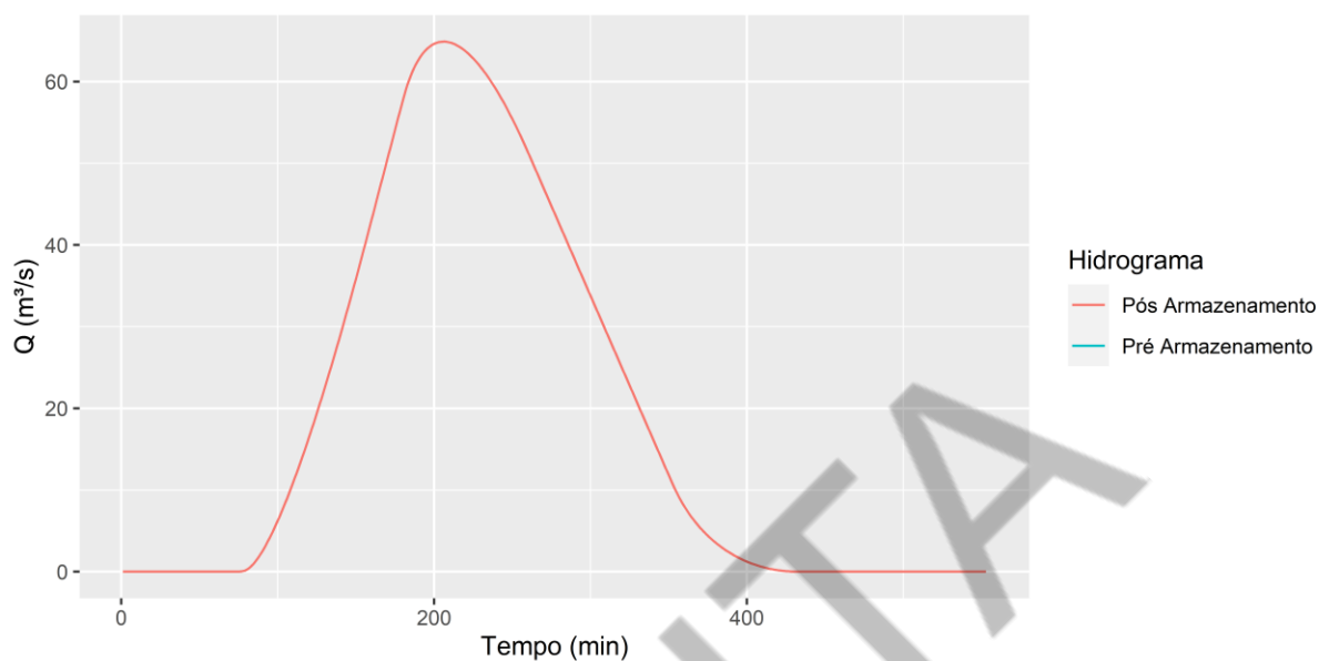
Figura 3 – Hidrogramas de Projeto SMB_01_03, com armazenamento e drenagem na fonte para expansão urbana de 5 anos.
