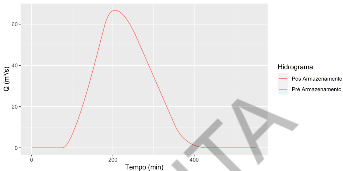
Figura 9 – Hidrogramas de Projeto SMB_01_03, com armazenamento e drenagem na fonte para expansão urbana de 15 anos.
