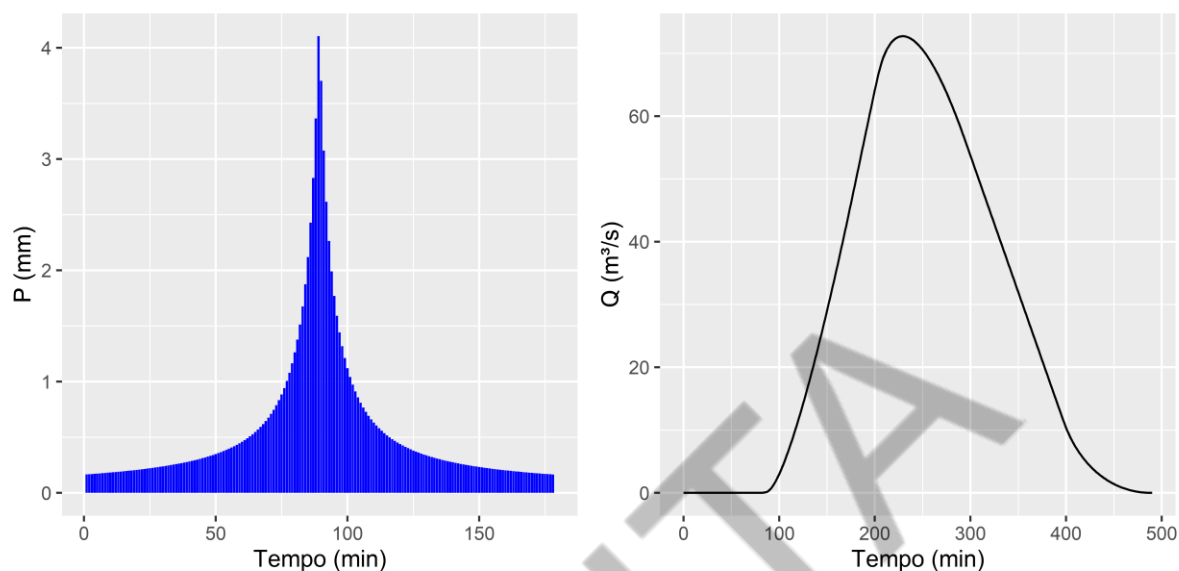
Figura 17 – Hietograma e Hidrograma de Projeto SMB_01_05, expansão urbana e drenagem na fonte de 30 anos.
