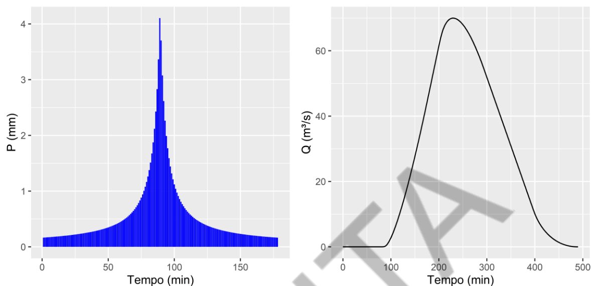
Figura 11 – Hietograma e Hidrograma de Projeto SMB_01_05, expansão urbana e drenagem na fonte de 15 anos.
