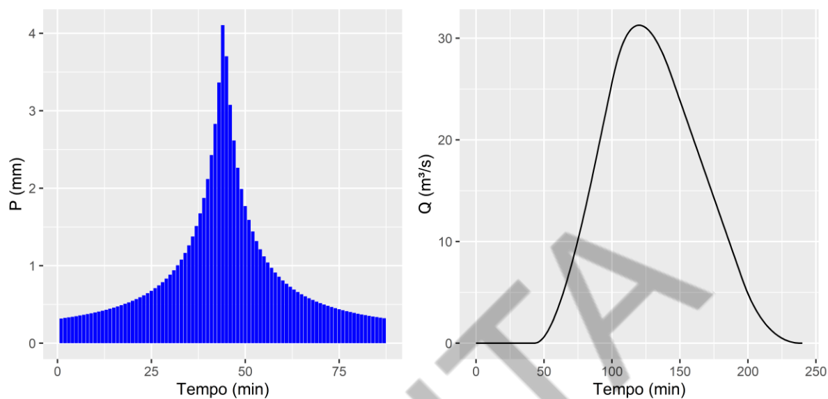
Figura 7 – Hietograma e Hidrograma de Projeto SMB_01_01, expansão urbana e drenagem na fonte de 15 anos.
