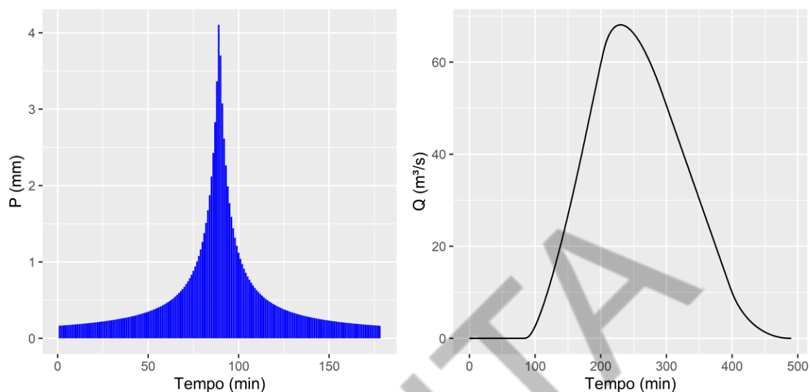
Figura 5 – Hietograma e Hidrograma de Projeto SMB_01_05, expansão urbana e drenagem na fonte de 5 anos.
