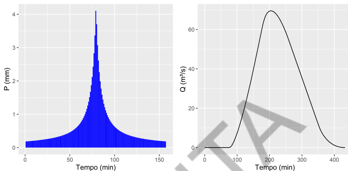
Figura 15 – Hietograma e Hidrograma de Projeto SMB_01_03, expansão urbana e drenagem na fonte de 30 anos.
