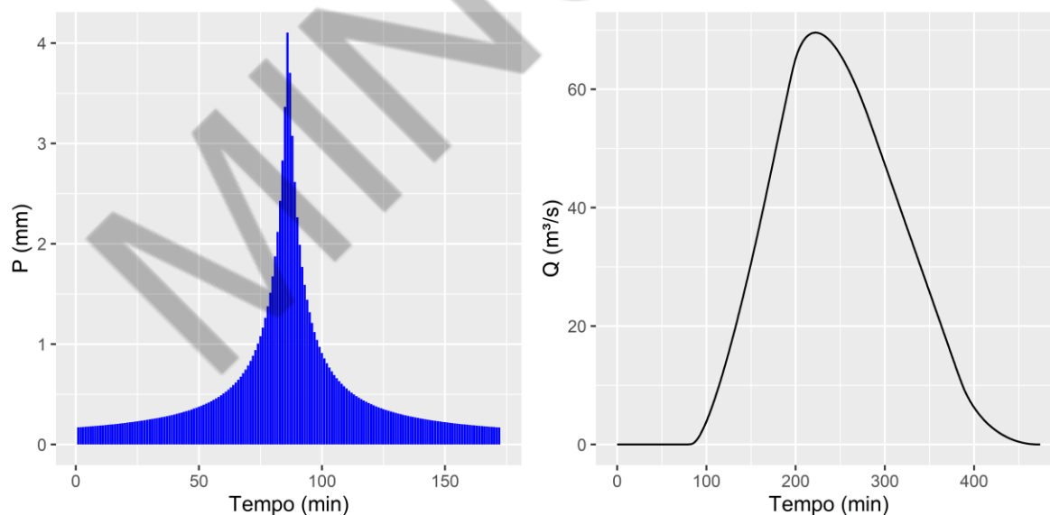
Figura 10 – Hietograma e Hidrograma de Projeto SMB_01_04, expansão urbana e drenagem na fonte de 15 anos.
