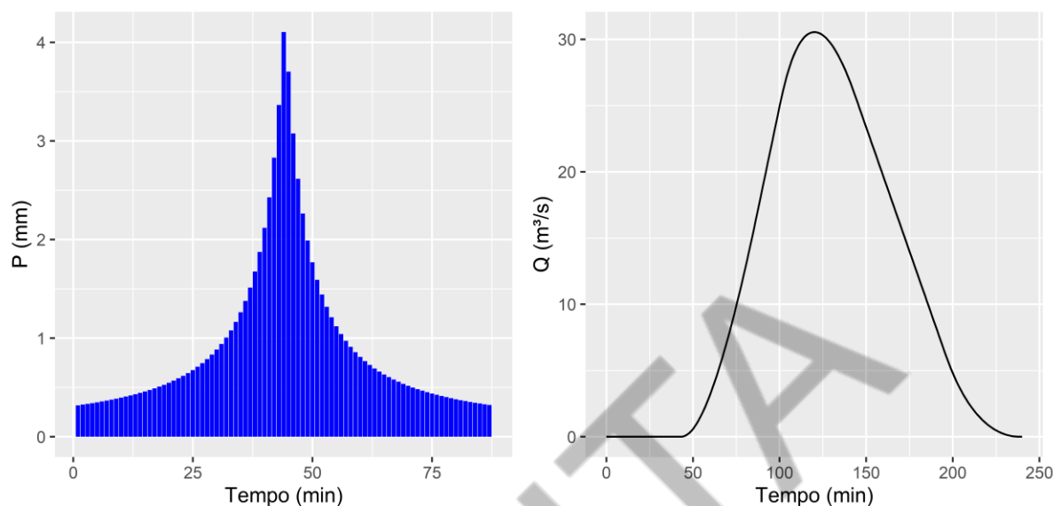
Figura 1 – Hietograma e Hidrograma de Projeto SMB_01_01, expansão urbana e drenagem na fonte de 5 anos.
