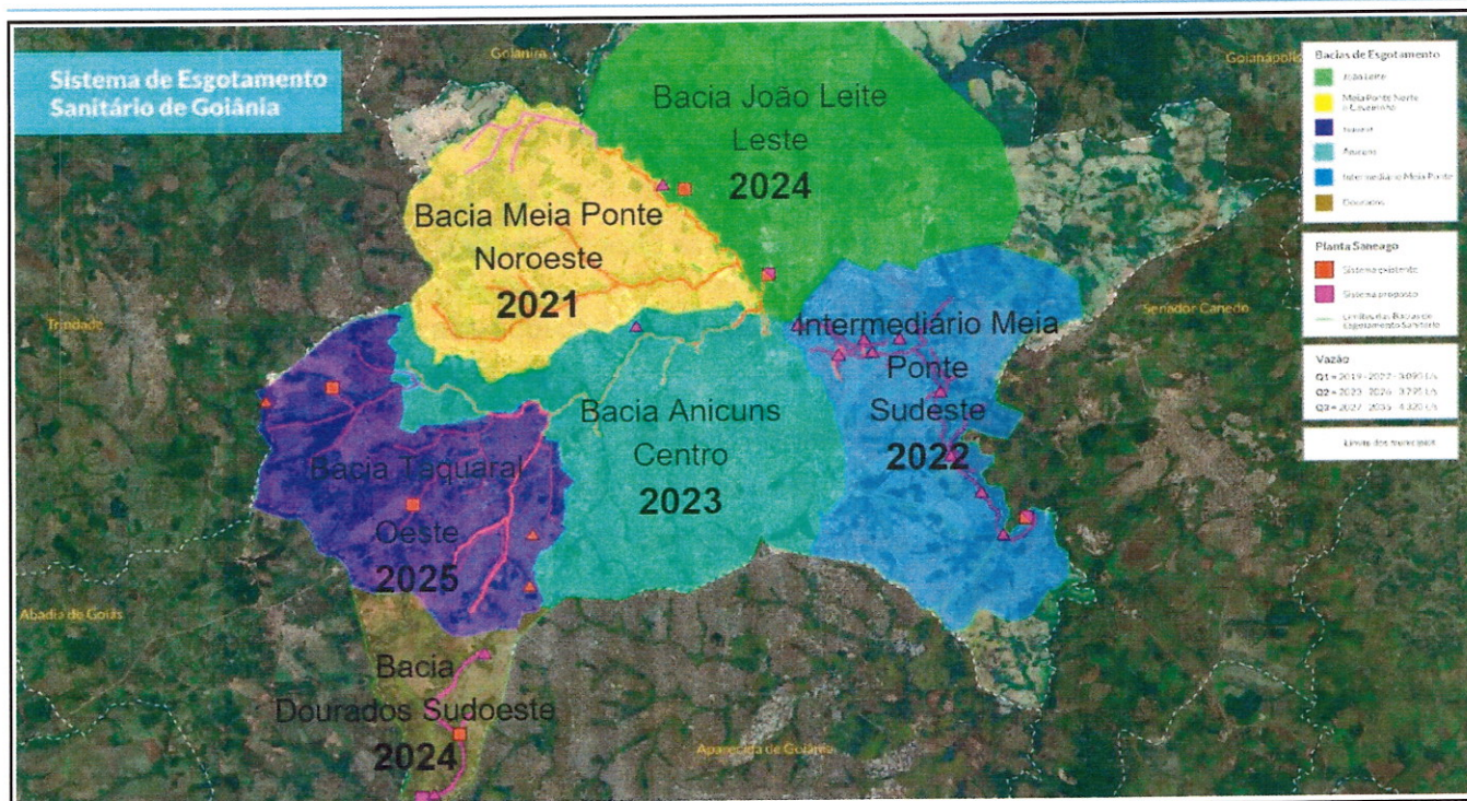
Figura 04. Mapa constante no PGP, denominado “Mapa 4 – Configuração esquemática das regiões e respectivos prazos de ampliação, reestruturação e melhoria do sistema de esgotamento sanitário.”
