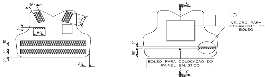
VISTA EXTERNA
