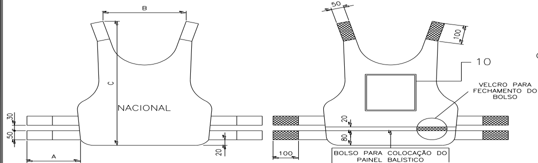
VISTA EXTERNA
