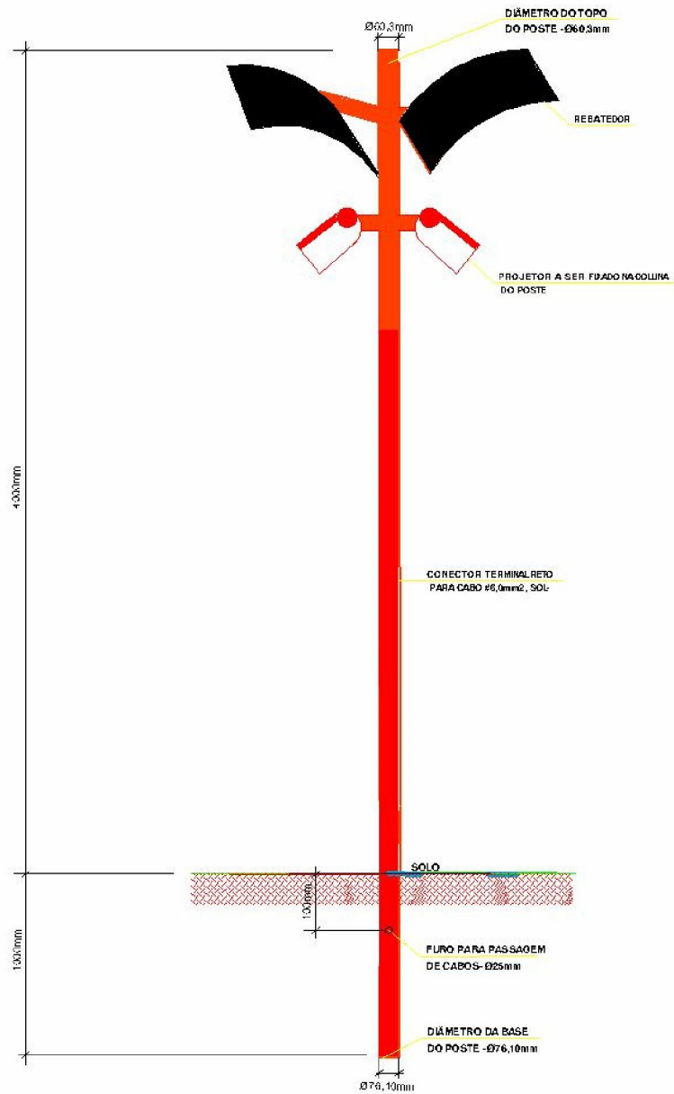
DETALHE CONSTRUTIVO DO POSTE SEM ESCALA
